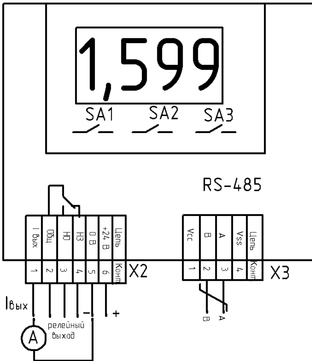
Рис. 26-8. Схема подключения датчика-реле давления ДРД-16.
